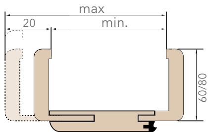
SCHEMAT OŚCIEŻNICY REGULOWANEJ
