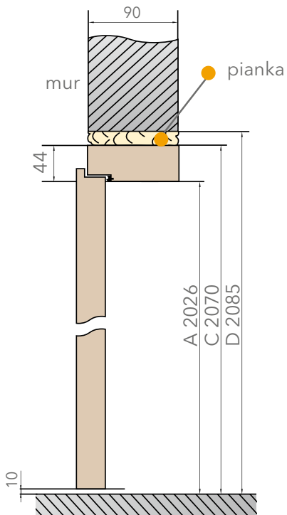
SCHEMAT OŚCIEŻNICY STAŁEJ
